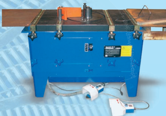
ohýbání betonářské oceli do průměru 32mm na stroji STEMA SPECIAL 42S
